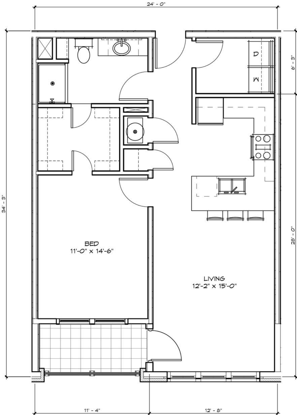
UNIT TYPE - 1.A 750 SF
