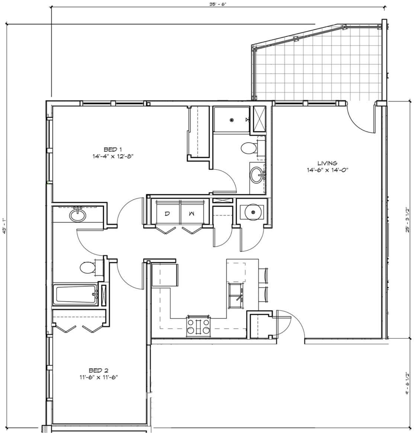
UNIT TYPE - 2.A 1000 SF
